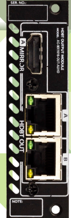
AC-MX1616-OUT-AUHD-HDBT
