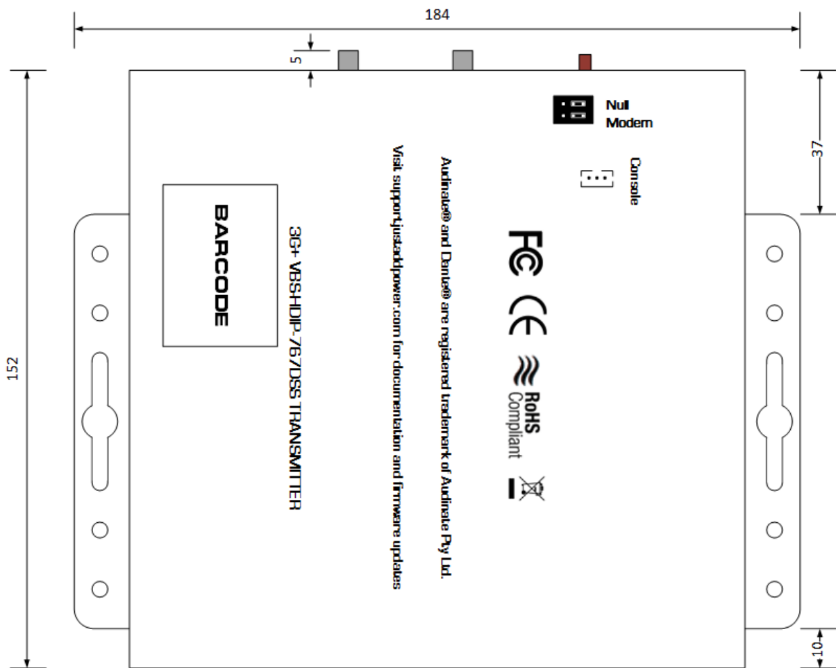
767DSS Bottom
