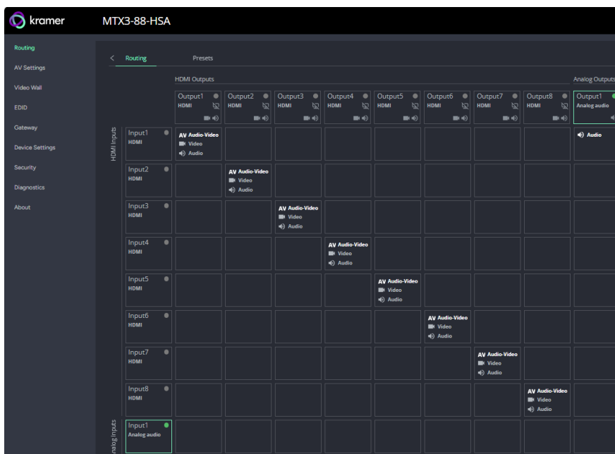
Figure 13: AV Routing Landing Page
