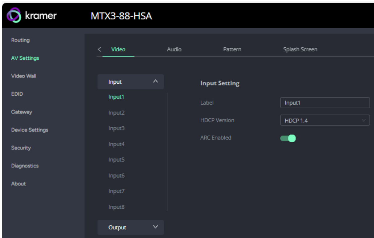
Figure 26: AV Settings Video Landing Page
